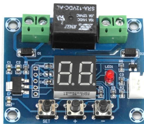
Рис.2 Внешний вид устройства Размеры платы: 43x52мм
