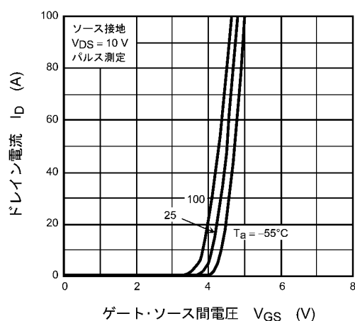
図 8.3 I_D - V_{GS}
