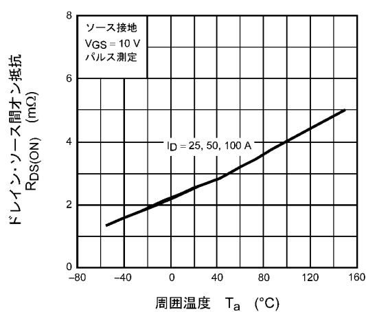
図 8.6 R_{DS(ON)} - T_a
