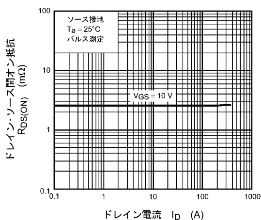
図 8.5 R_{DS(ON)} - I_D
