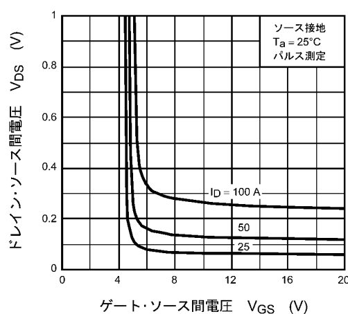
図 8.4 V_{DS} - V_{GS}
