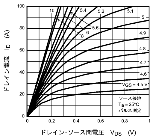
図 8.1 I_D - V_{DS}
