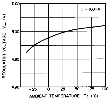
Fig.6 レギュレータ電圧-温度特性
