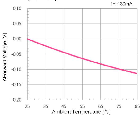
▪ V_F vs. Temp.
