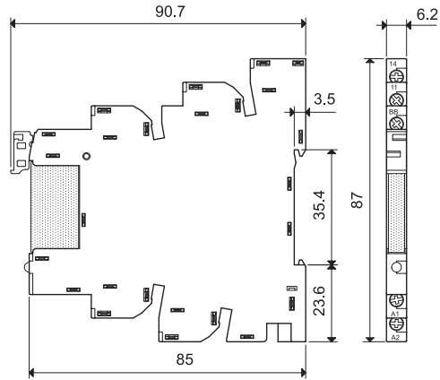
39.40 39.41 Винтовой зажим
