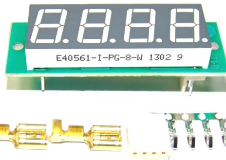
Внешний вид устройства (размер платы 22x63мм)
