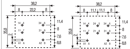
62.22 - 0300 Вид сбоку
