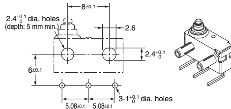
<PCB Cutout Dimensions (Reference)>
